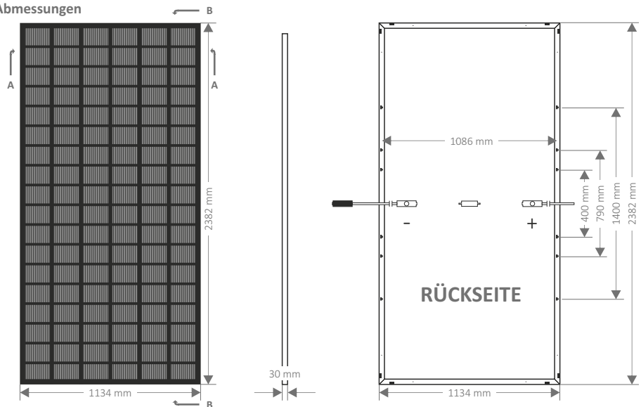
Abmessungen
